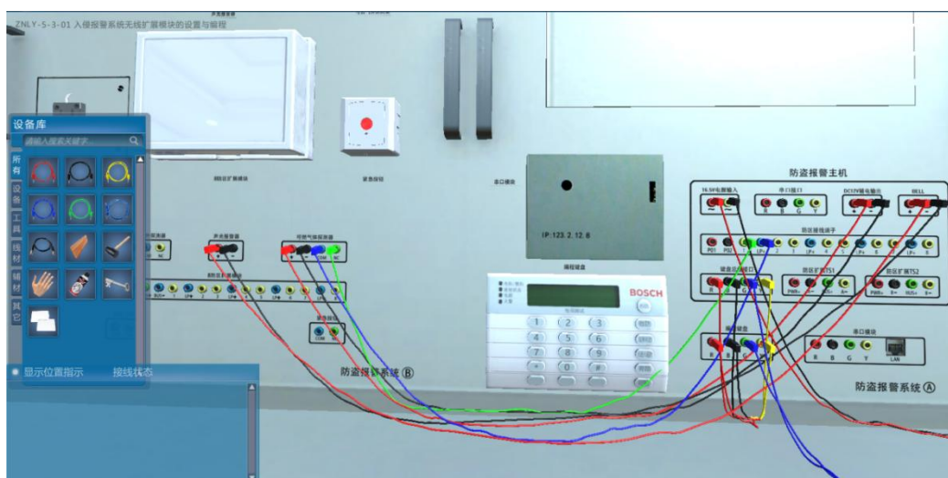
接线图
